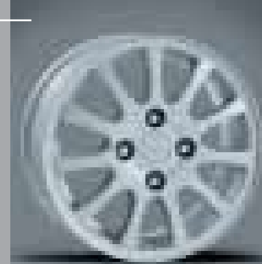
Leichtmetallfelge - 6J X 15" 11 Speichen MR914439 Nabendeckel - MR316517 Radmuttern - MB579290
